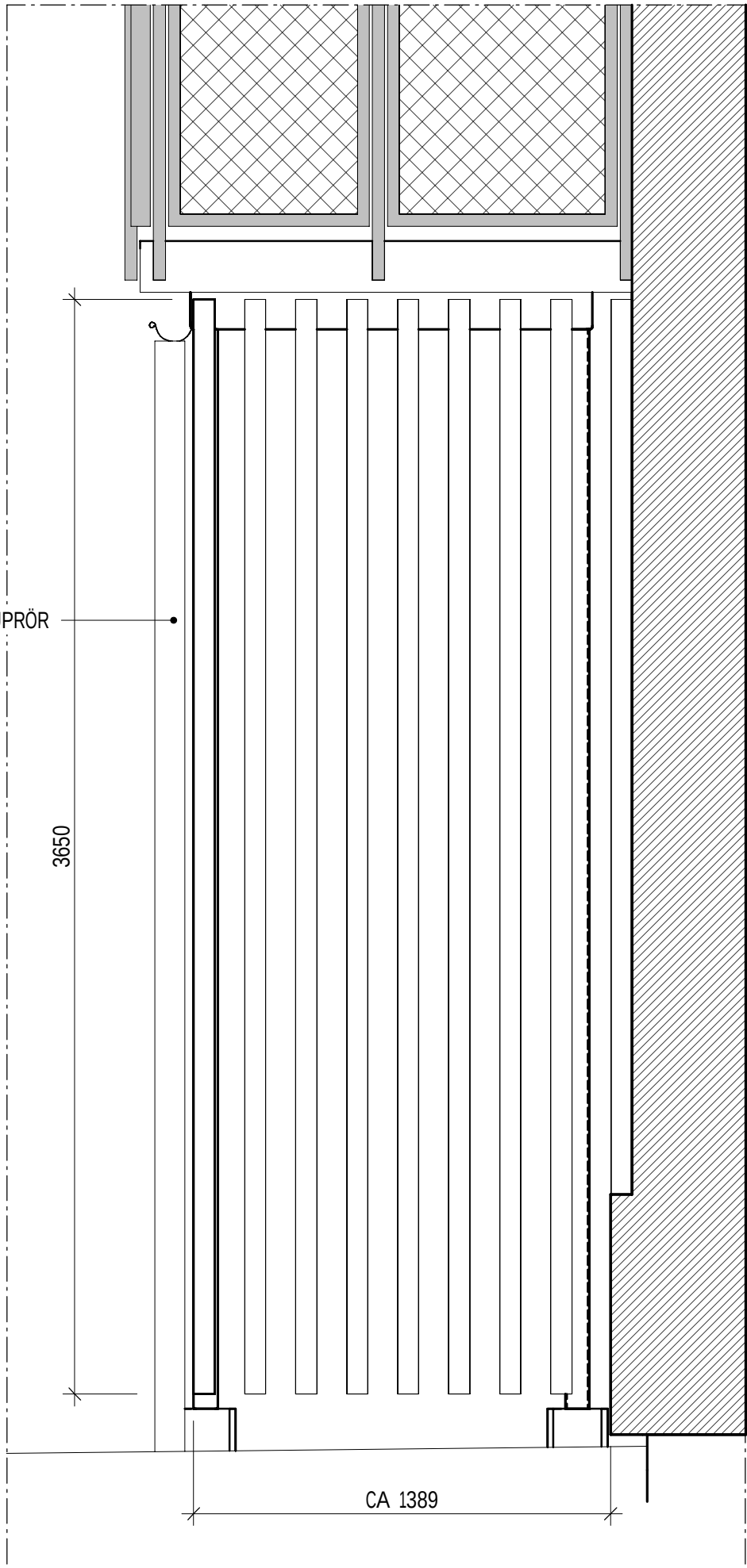
Elevation - SPALJÉ 3b 1 : 20
