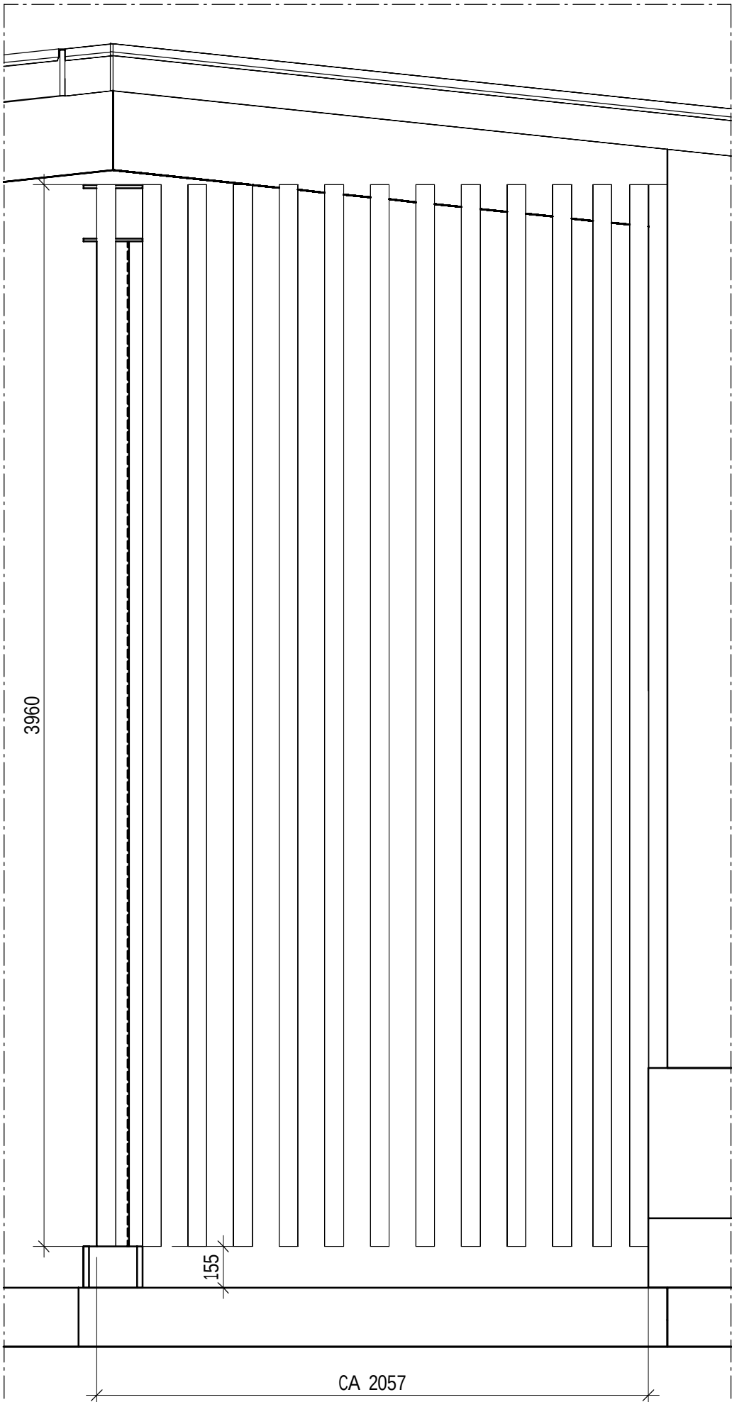
Elevation - SPALJÉ 2 1 : 20
