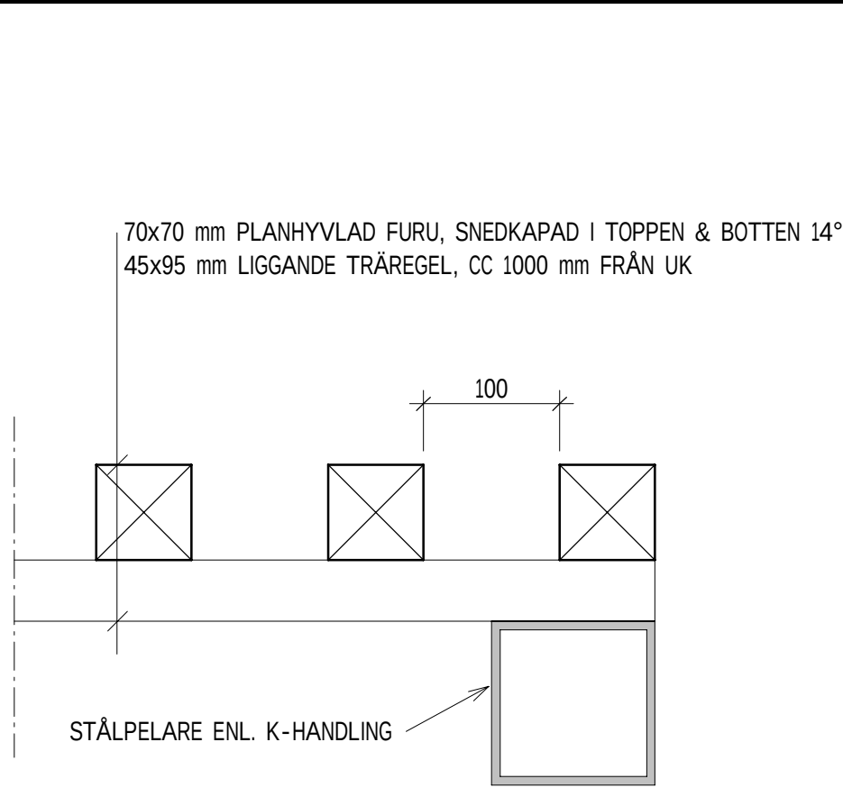
HORISONTAL PRINCIPDETALJ SPALJÉ 1 1 : 5
