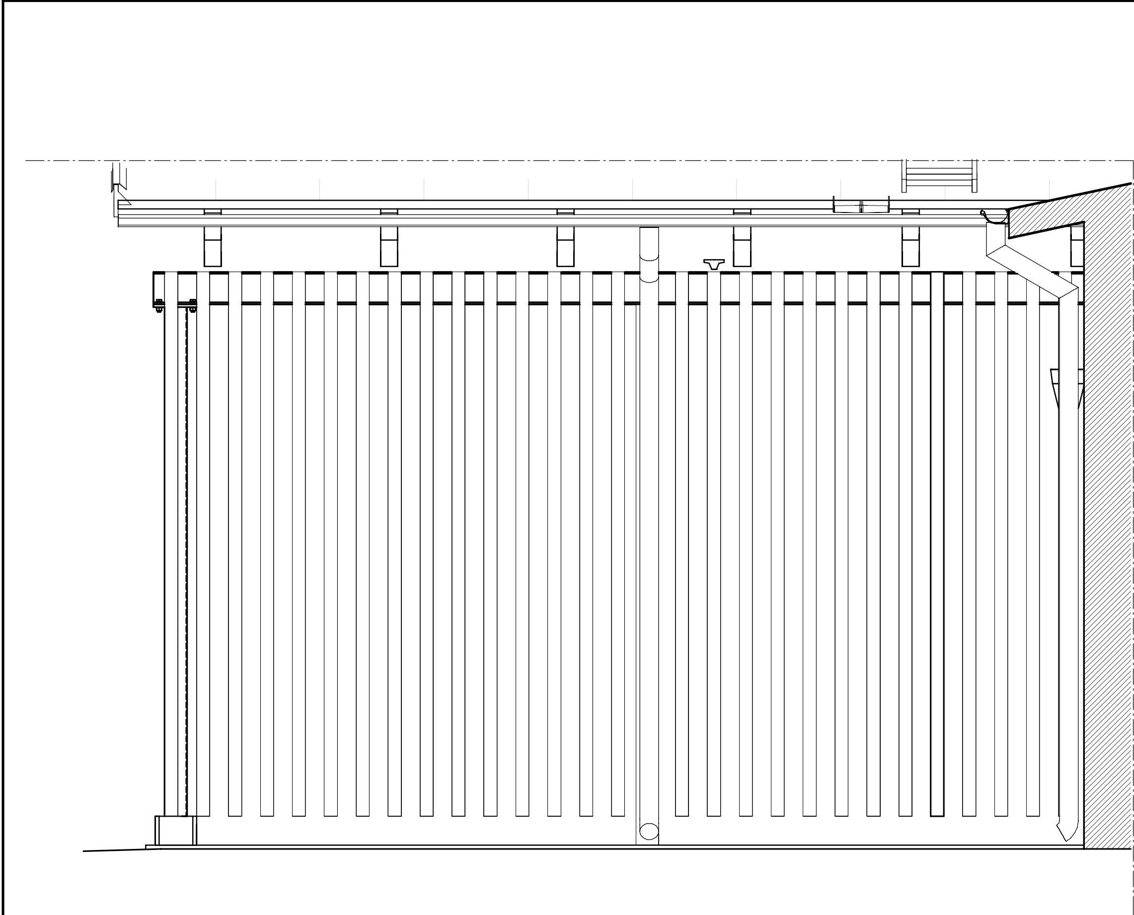
Elevation - SPALJÉ 1 1 : 20
