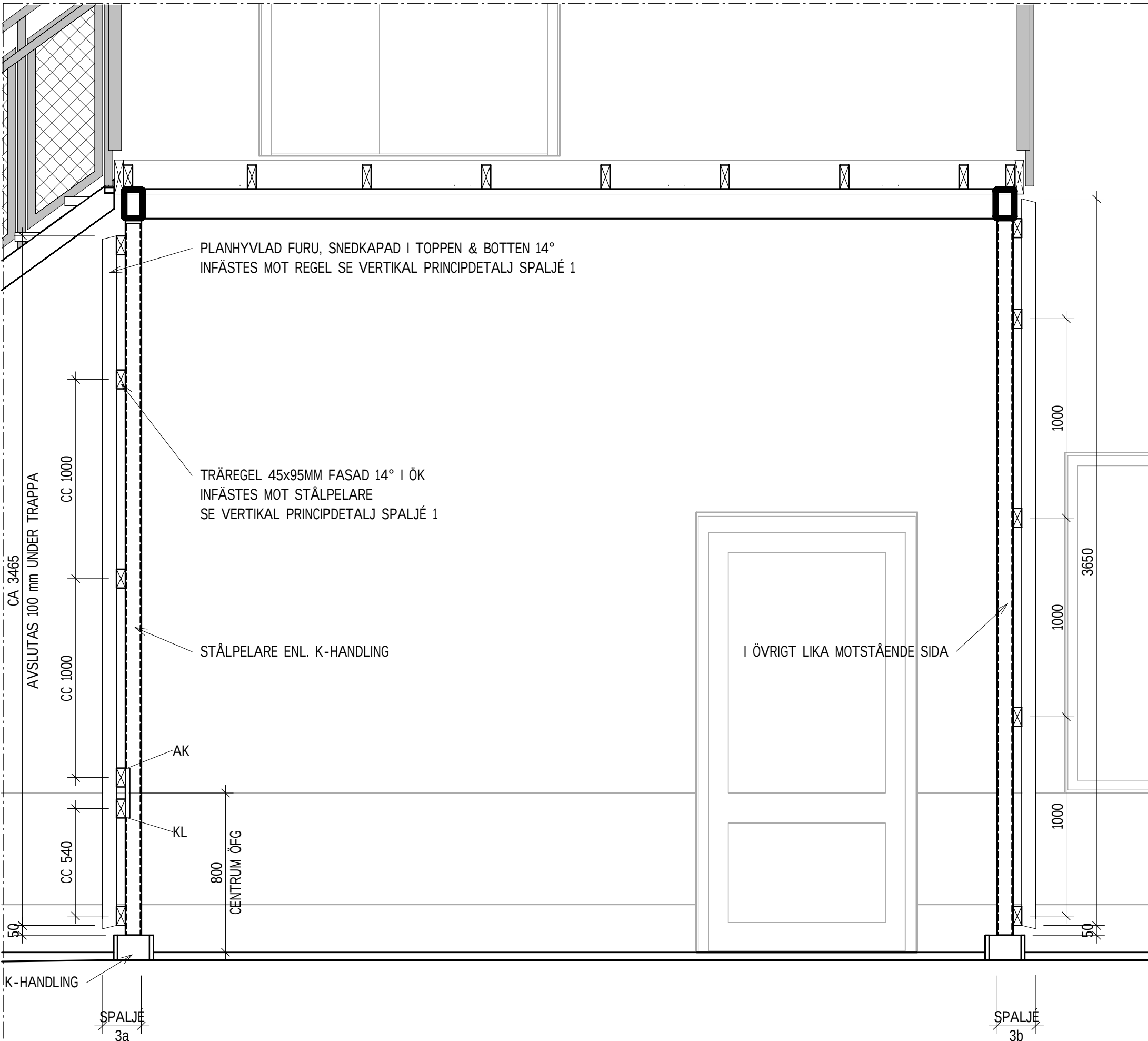
SPALJÉ 3 - SEKTION 1 : 20
