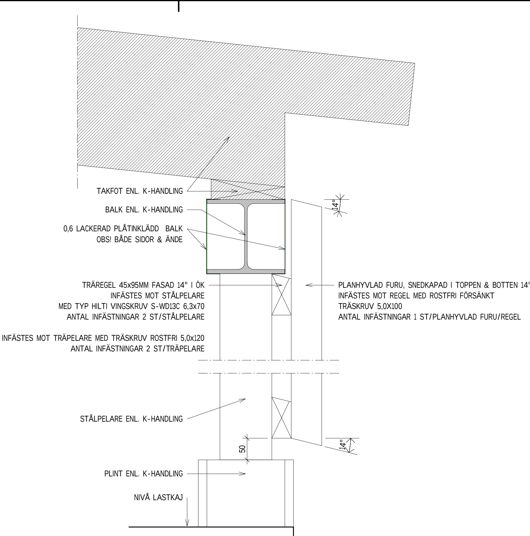
VERTIKAL PRINCIPDETALJ SPALJÉ 1 1 : 5
